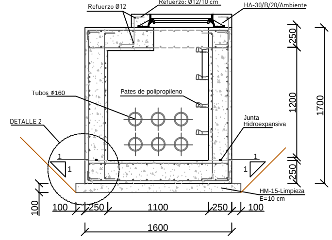
Sección B-B'
