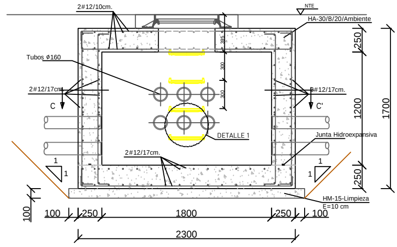
Sección A-A'
